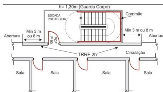
Figura 20 - Escada aberta externa
