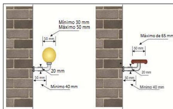
Figura 23 - Pormenores de corrimãos
