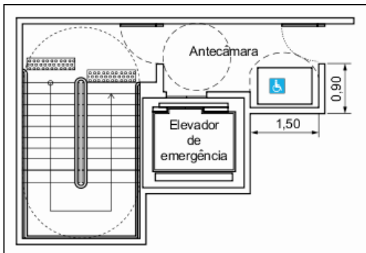
Figura 16: Escada enclausurada à prova de fumaça, com área para pessoas com deficiência.
