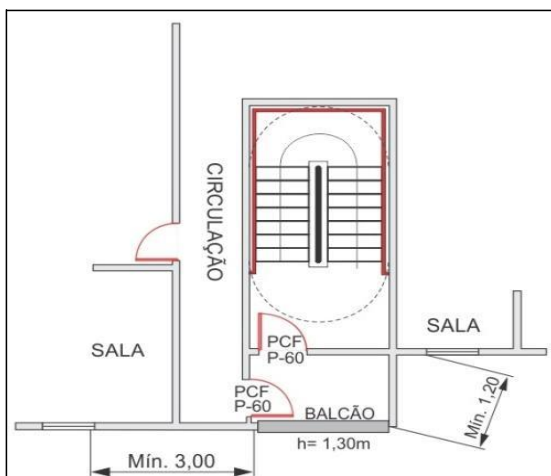
Figura 19 - Escada enclausurada do tipo PF ventilada por balcão
