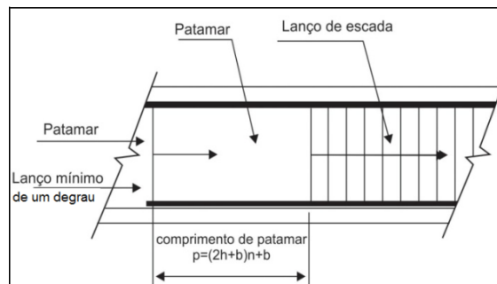
Figura 6 - Lanço mínimo e comprimento de patamar
