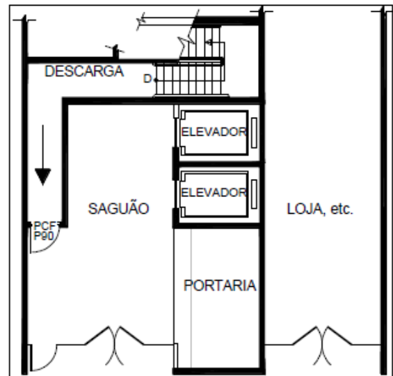
Figura 26 - (ilustrativa) Descarga através de hall térreo não enclausurado.
