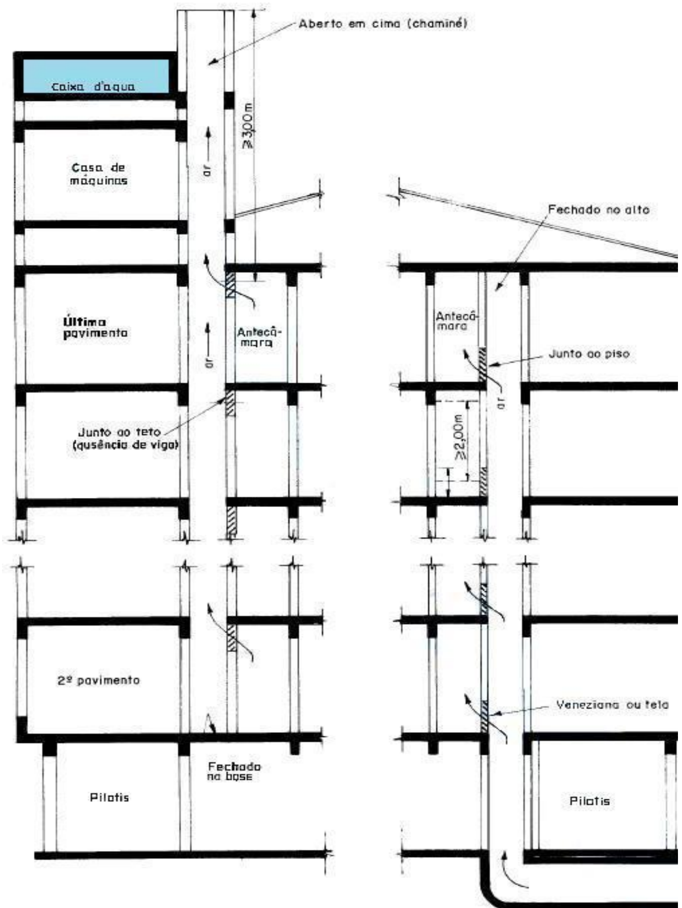
Figura 18 - Exemplos de dutos de ventilação (corte AB e corte CD)
