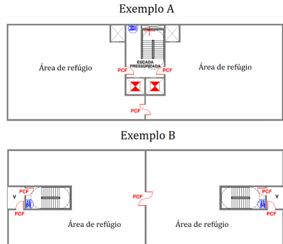
Figura 25: Exemplos esquemáticos de áreas de refúgio (ilustrativo).
