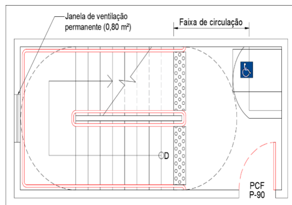
Figura 7 - Escada enclausurada protegida
