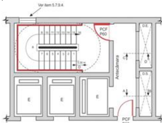
Figura 17- Escada enclausurada à prova de fumaça
