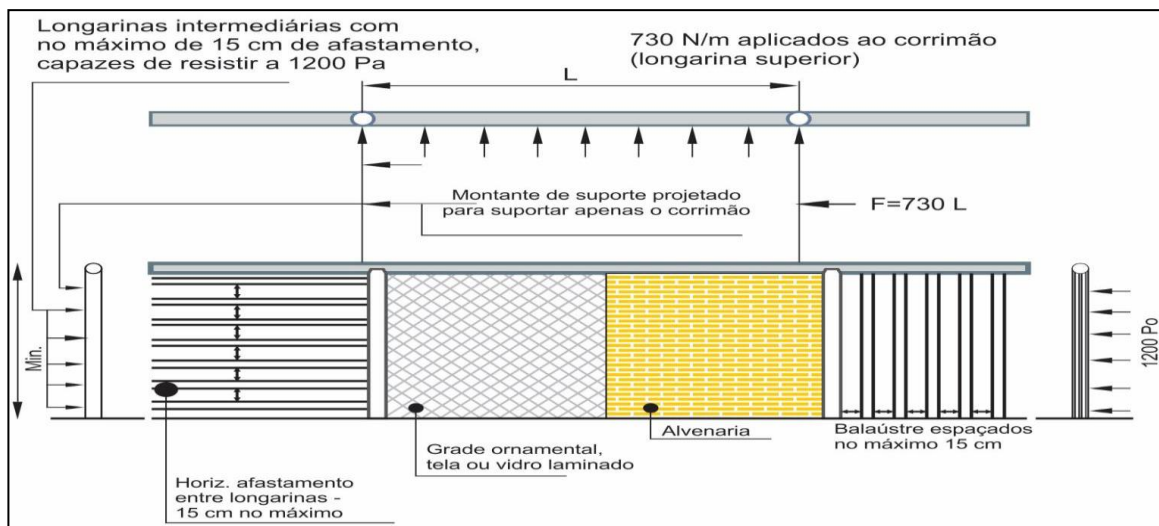
Figura 24 - Pormenores construtivos da instalação de guardas e as cargas a que elas devem resistir
