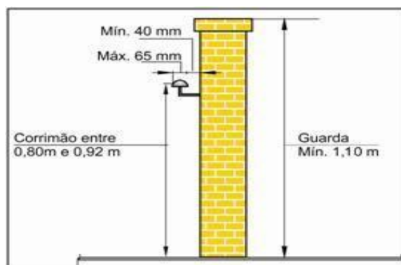
Figura 22 - Dimensões de guardas e corrimãos
