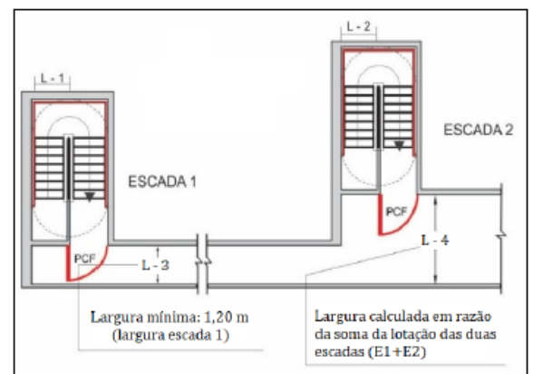
Figura 27 – Dimensionamento de corredores de descarga.
