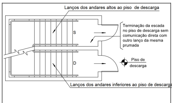
Figura 3 - Segmentação das escadas no piso da descarga
