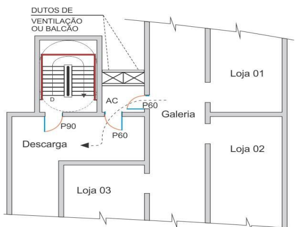
Figura 28 - Acesso de galeria comercial à descarga.
